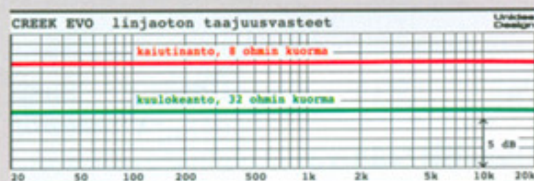
Taajuusvasteet
