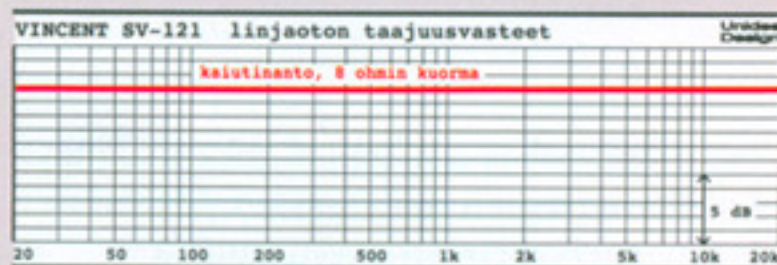
Taajuusvasteet
